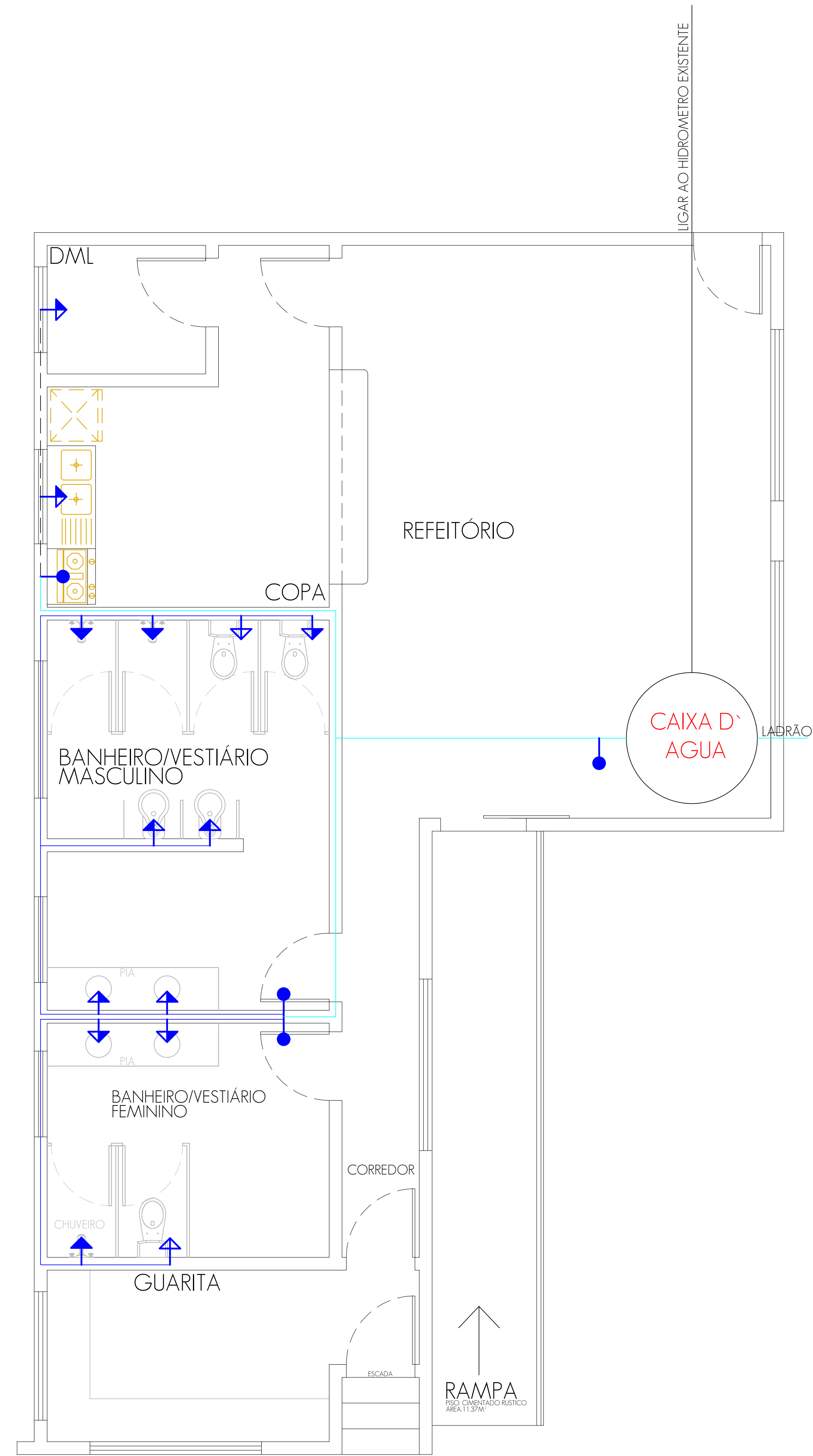
PLANTA BAIXA HIDRAULICA Escala 1/35
